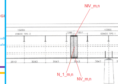
Giunto bullonato tra conci m e n, lato 1 (Sx)
